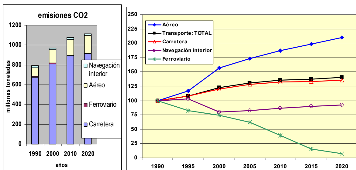
Gráfico 3-2: Evolución esperada de las emisiones de CO 2 , por modo de transporte (1990 = 100)
