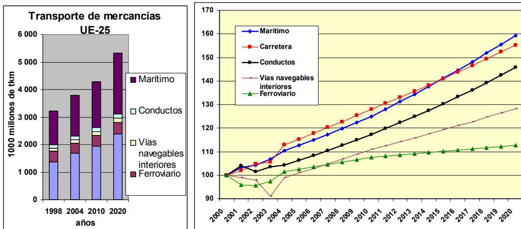
Gráfico 2-1: Crecimiento esperado de la actividad de transporte de mercancías, por modo de transporte (2000=100)
