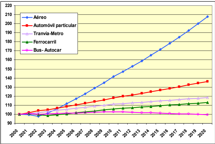
Gráfico 2-2: Crecimiento esperado de la actividad de transporte de viajeros, por modo de transporte (2000=100)
