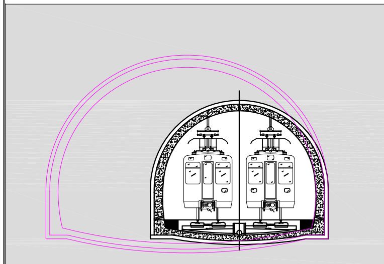
SECCIÓN TIPO 4
