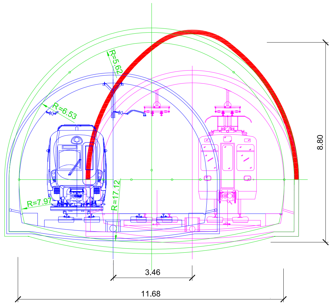
SECCIÓN TIPO 3
