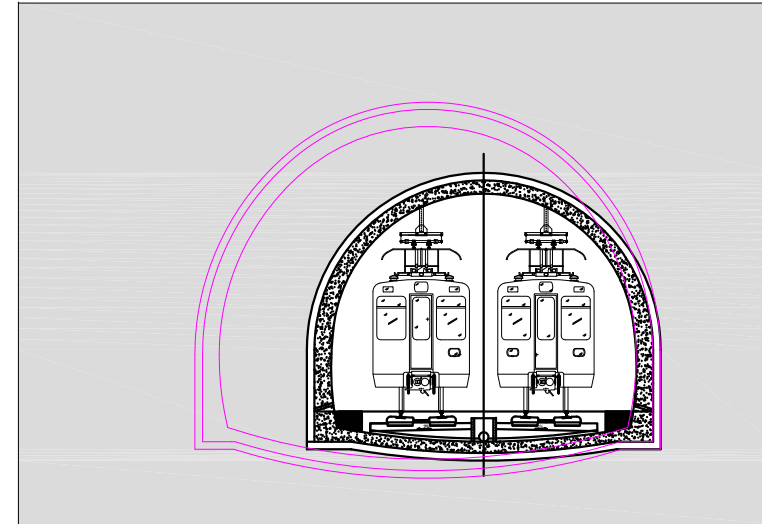
SECCIÓN TIPO 3
