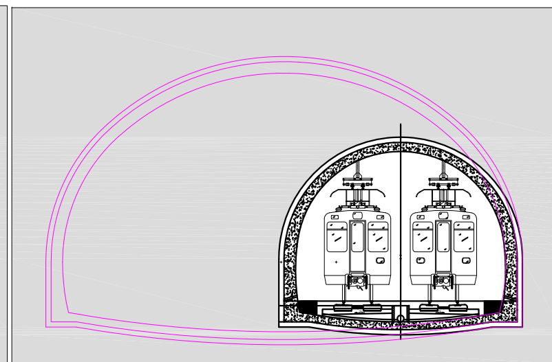
SECCIÓN TIPO 5
