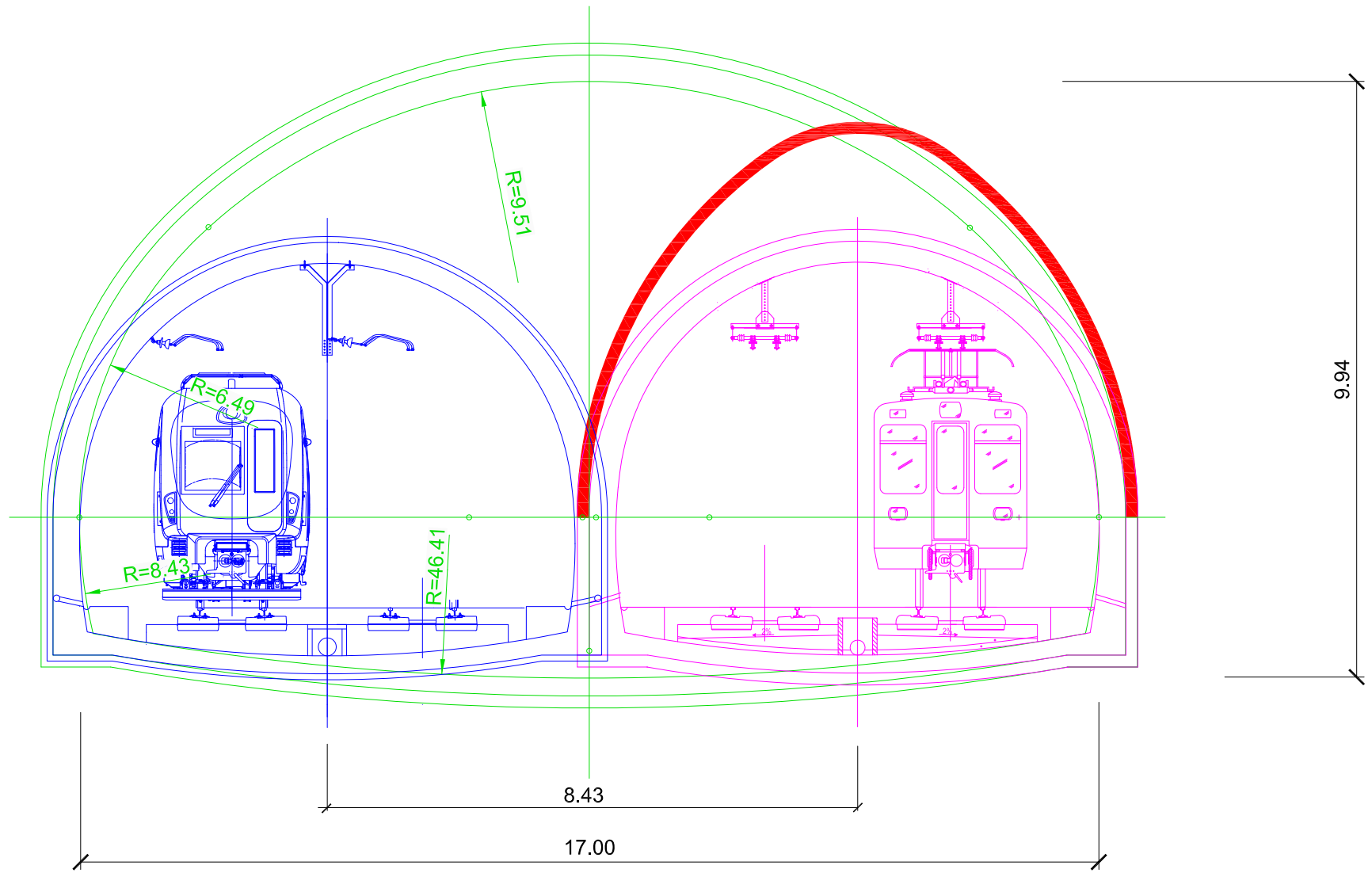
SECCIÓN TIPO 5
