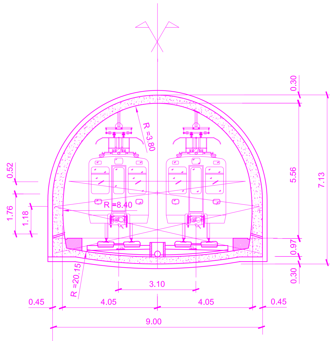
SECCIÓN TIPO 1
