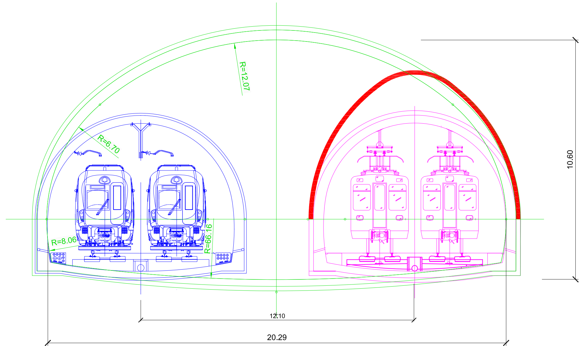
SECCIÓN TIPO 6
