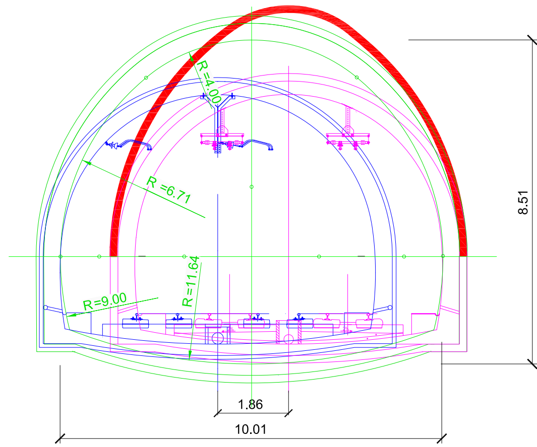
SECCIÓN TIPO 2
