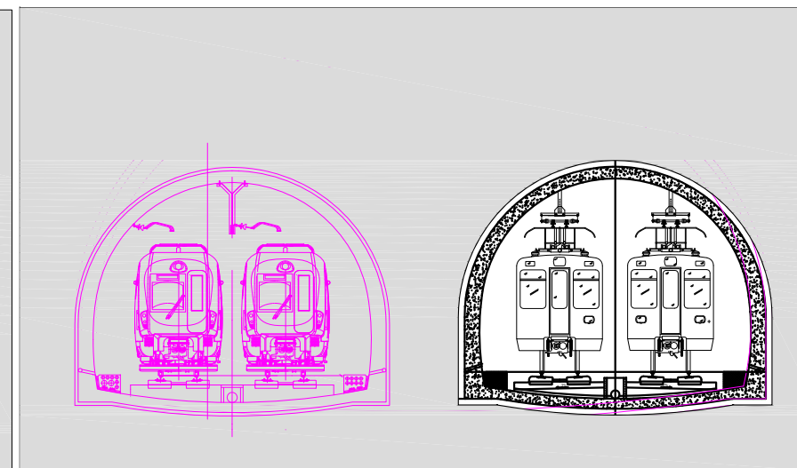
SECCIÓN TIPO 6
