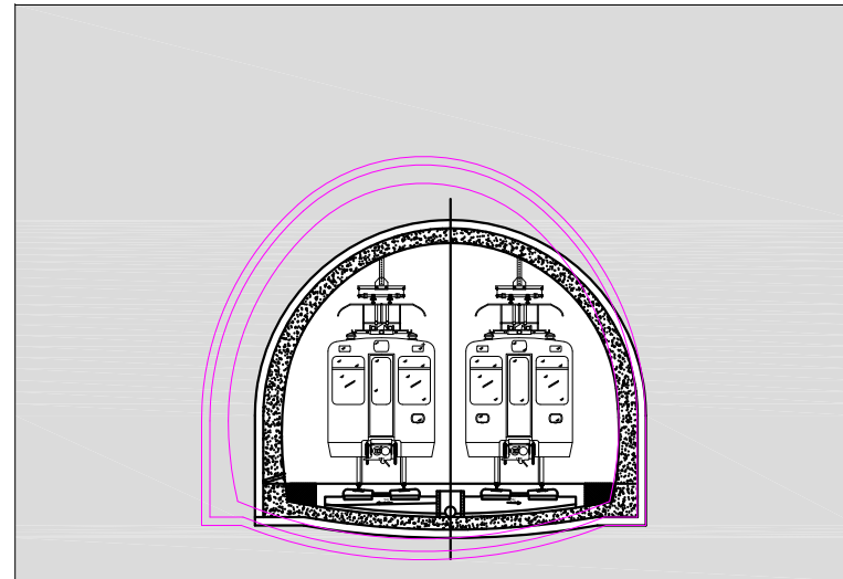
SECCIÓN TIPO 2
