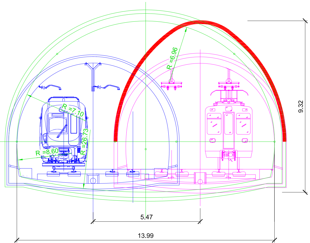
SECCIÓN TIPO 4
