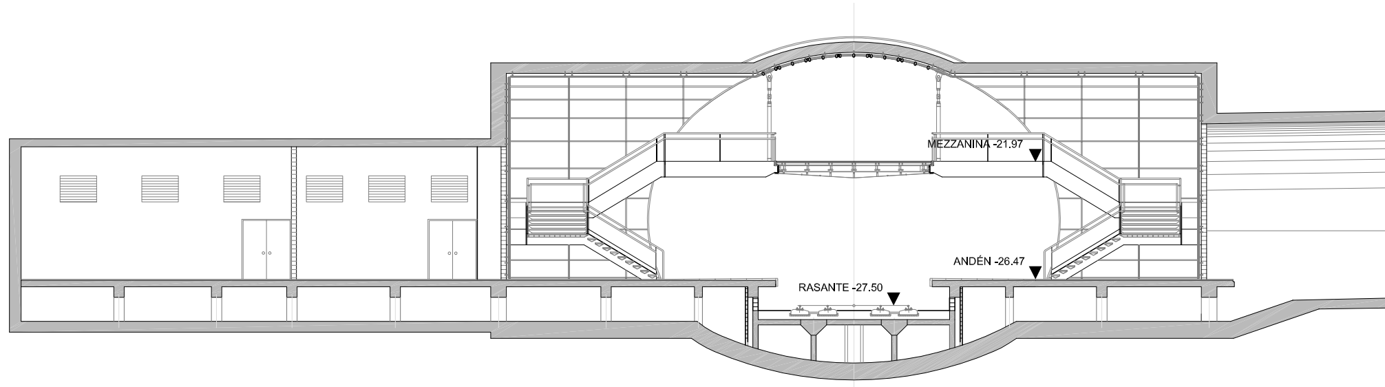
SECCIÓN A-A E(A1): 1/100
