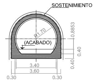
SECCIÓN B-B E(A1): 1/100
