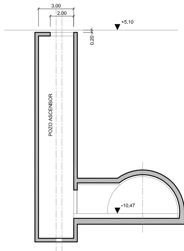
SECCIÓN A-A E(A1): 1/100
