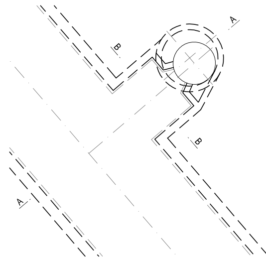
PLANTA NIVEL DE SUPERFICIE +5.10 E(A1): 1/100
