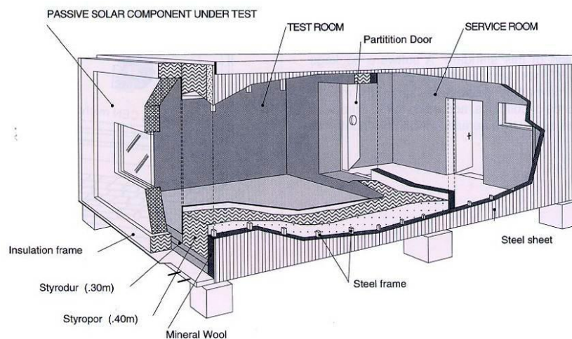
Figura 2.6 - Estructura general de una célula de ensayos PASLINK.
