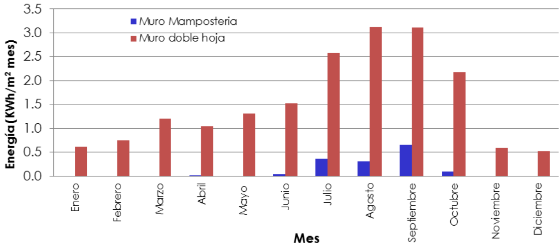
Figura 4.3. Ganancias Térmicas [kWh/m 2 mes] a lo largo del año en los dos cerramientos existentes estudiados
