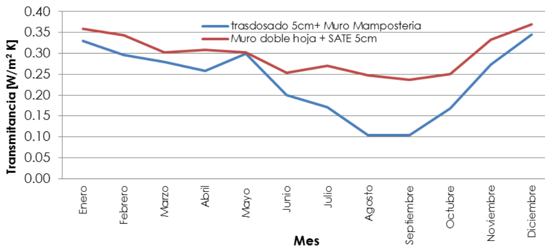
Figura 4.4. Transmitancia dinámica [W/m²K] a lo largo del año en los dos cerramientos rehabilitados estudiados
